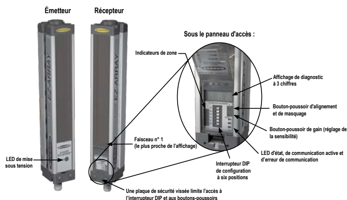
Illustration 3. Émetteur et récepteur
