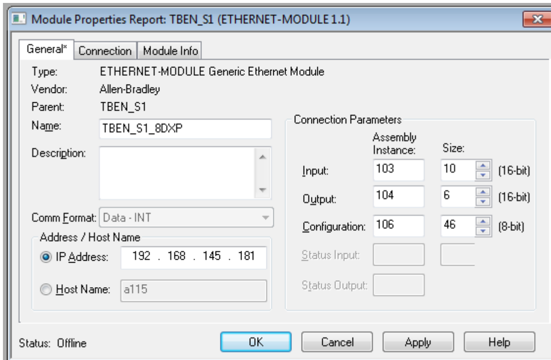
Abb. 67: Modulnamen und IP-Adresse einstellen
