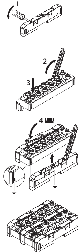
Abb. 9: Modulgruppen für die Montage auf Hutschiene (TS35) bilden
