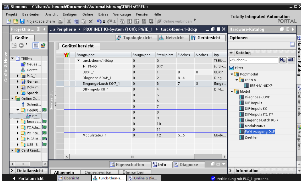
Abb. 41: TIA-Portal – TBEN-S1-8DXP – Belegung der Slots und Subslots
