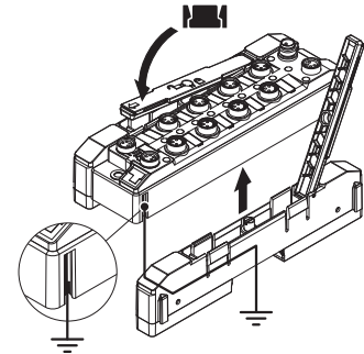
Abb. 17: Erdung der Verbindertbnn-s0-drs
