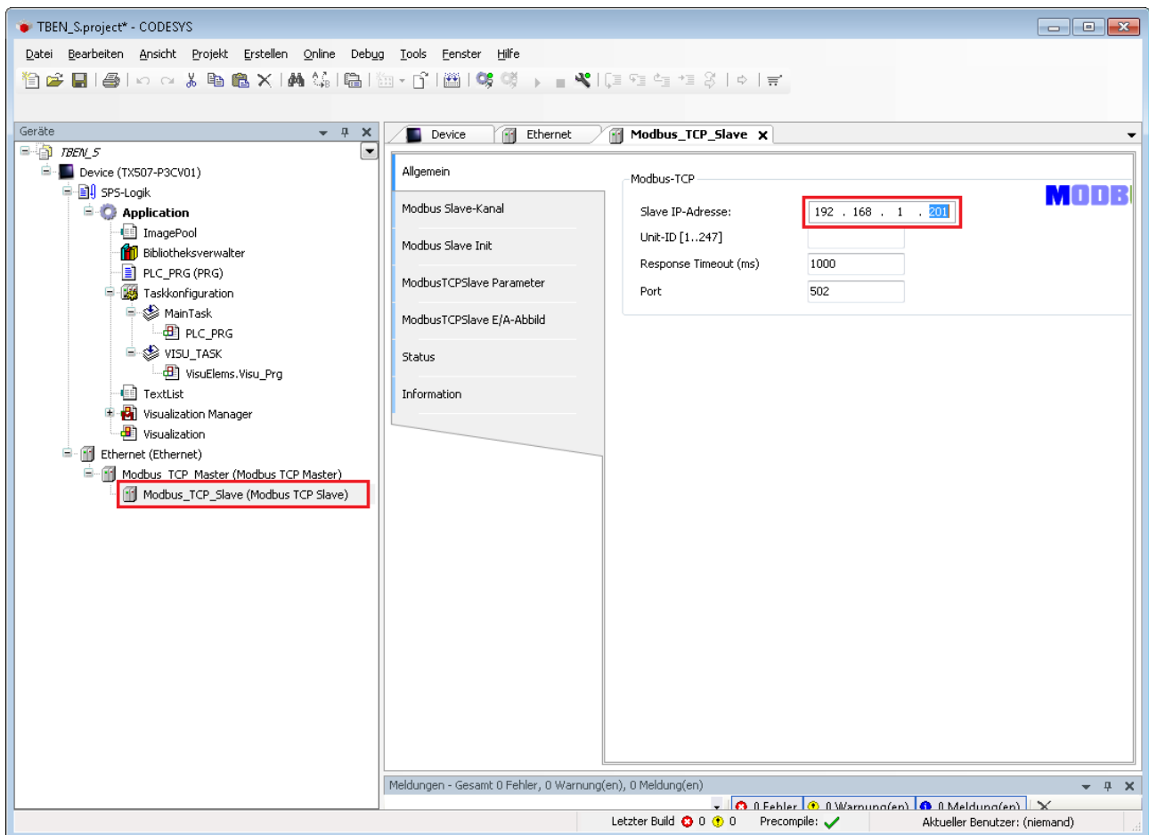
Abb. 58: Modbus-Slave – IP-Adresse einstellen
