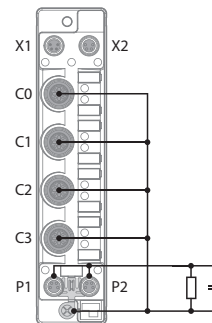
Abb. 13: Ersatzschaltbild, Schirmkonzept – TBEN-S2-Digitalmodule
