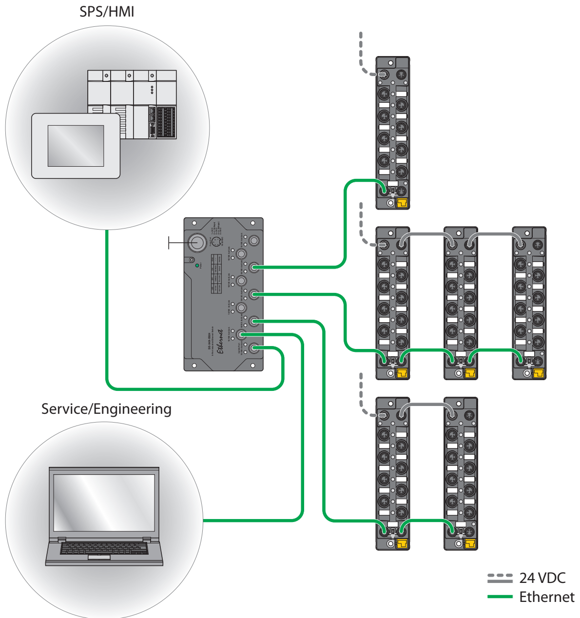
Abb. 4: Netzwerkstruktur, Beispiel 1
