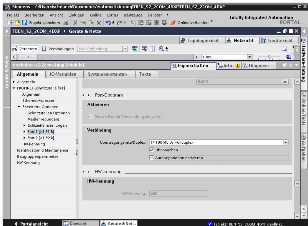
Abb. 42: TIA-Portal – Port-Einstellung für FSU
