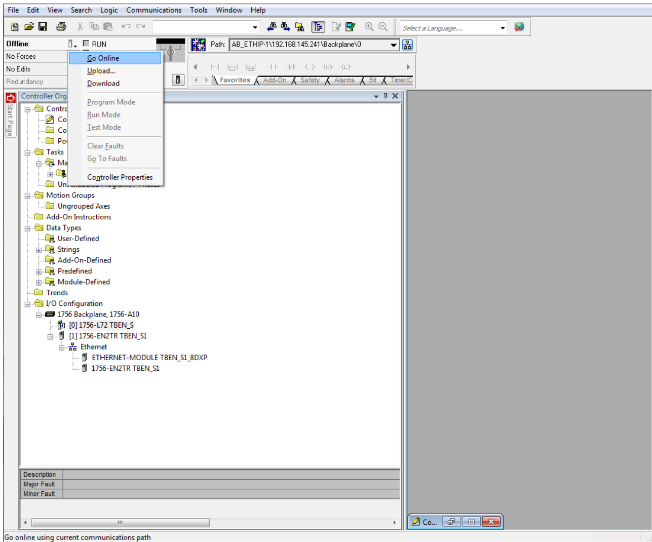
Abb. 71: Gerät online verbinden
