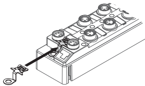
Abb. 19: Erdungsspanne montieren
