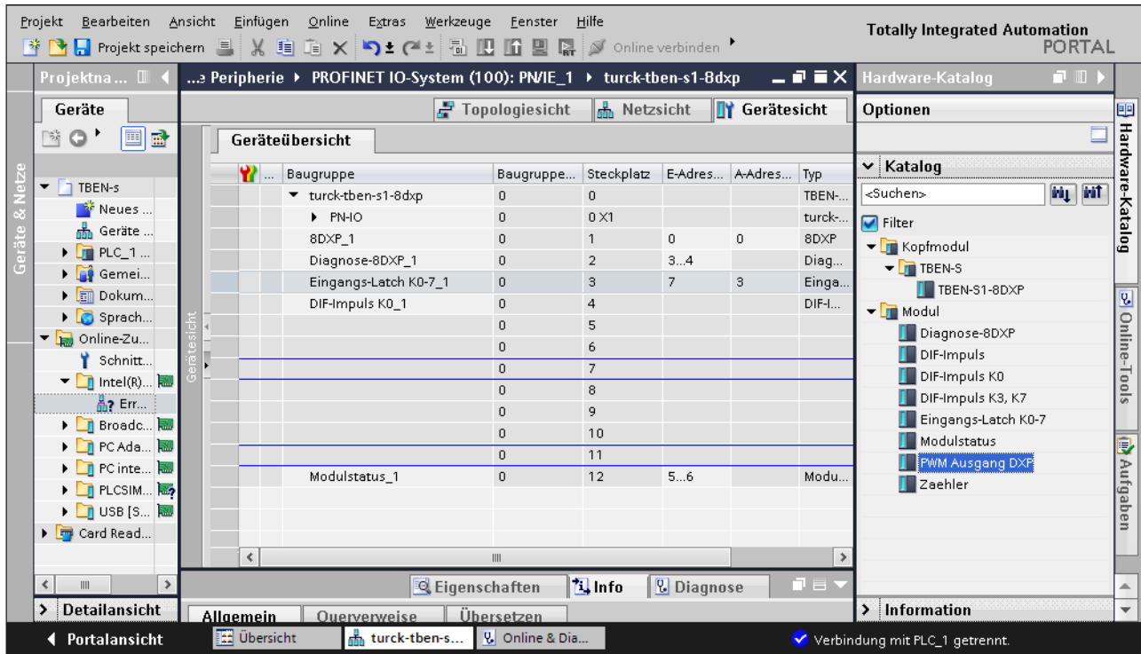
Abb. 47: Steckplätze des Geräts konfigurieren
