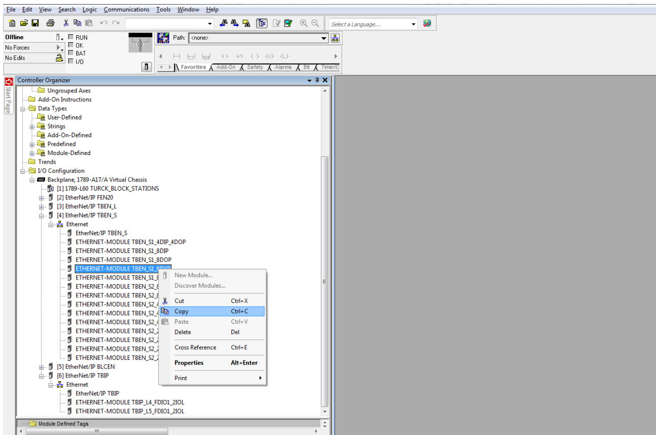
Abb. 65: RSLogix – Geräteeintrag aus Catalog-Datei kopieren
