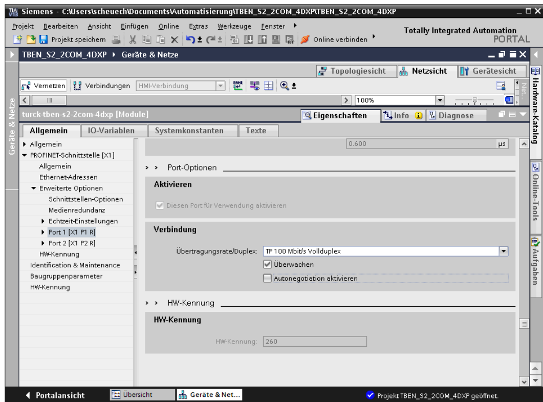
Abb. 43: TIA-Portal – Priorisierter Hochlauf, Aktivierung am I/O-Gerät
