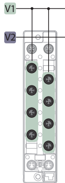
Abb. 24: Versorgung TBEN-S1-8DIP/-8DIP-D
