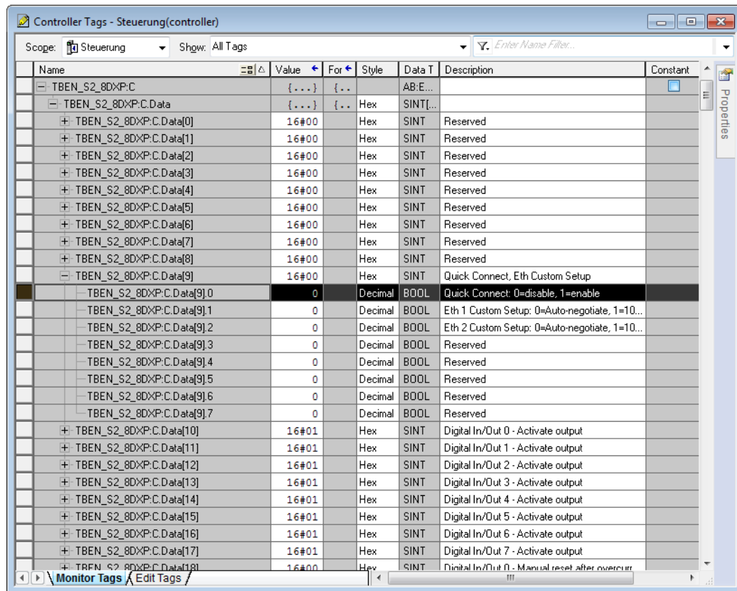
Abb. 62: QuickConnect in RSLogix konfigurieren
