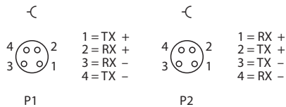
Abb. 21: Ethernet-Anschlüsse – Pinbelegung P1 und P2
