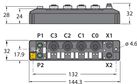
Abb. 2: TBEN-S2-... – Abmessungen
