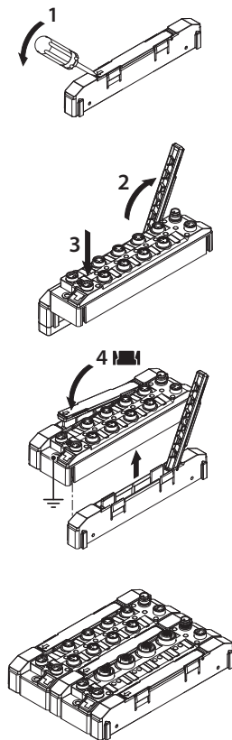
Abb. 8: Modulgruppen für die Montage auf Montageplatte bilden
