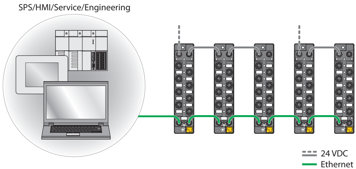
Abb. 6: Netzwerkstruktur, Beispiel 3
