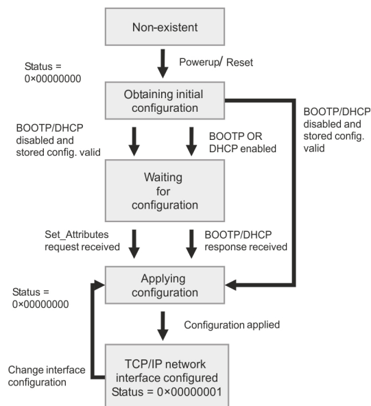
Abb. 64: TCP/IP Objektstatus-Diagramm (gemäß CIP Spez., Vol.2, Rev. 1.1)
