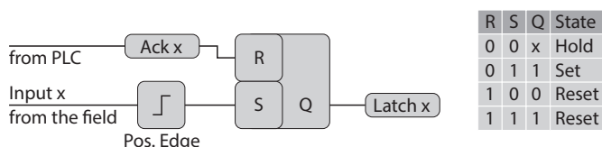
Abb. 3: Input-Latch-Funktion
