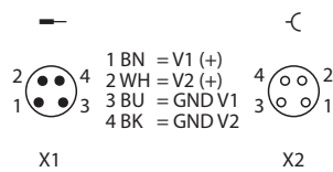
Abb. 23: Pinbelegung Versorgungsspannungs-Anschlüsse
