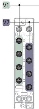
Abb. 26: Versorgung TBEN-S1-4DIP-4DOP/ TBEN-S1-8DXP
