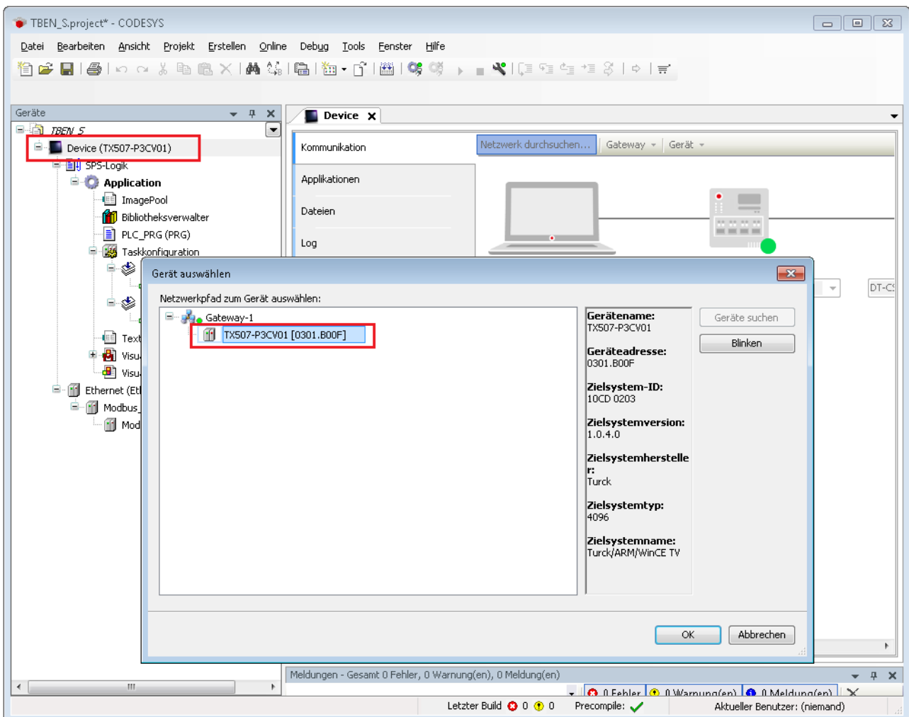
Abb. 56: Netzwerk-Schnittstelle zum Modbus-Master einrichten
