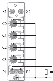
Abb. 14: Ersatzschaltbild, Schirmkonzept – TBEN-S2-Analogmodule
