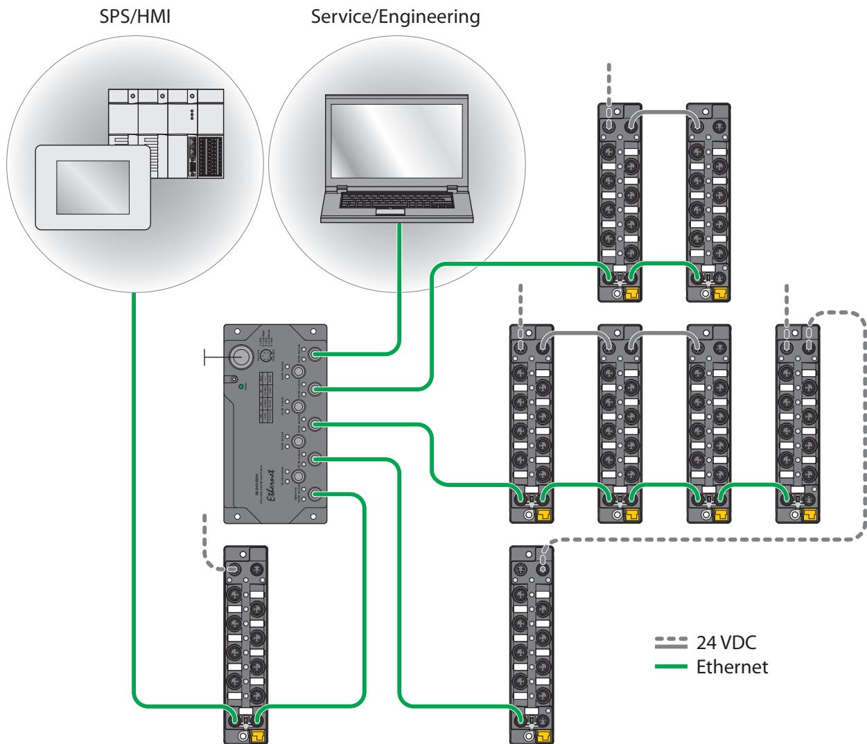
Abb. 5: Netzwerkstruktur, Beispiel 2
