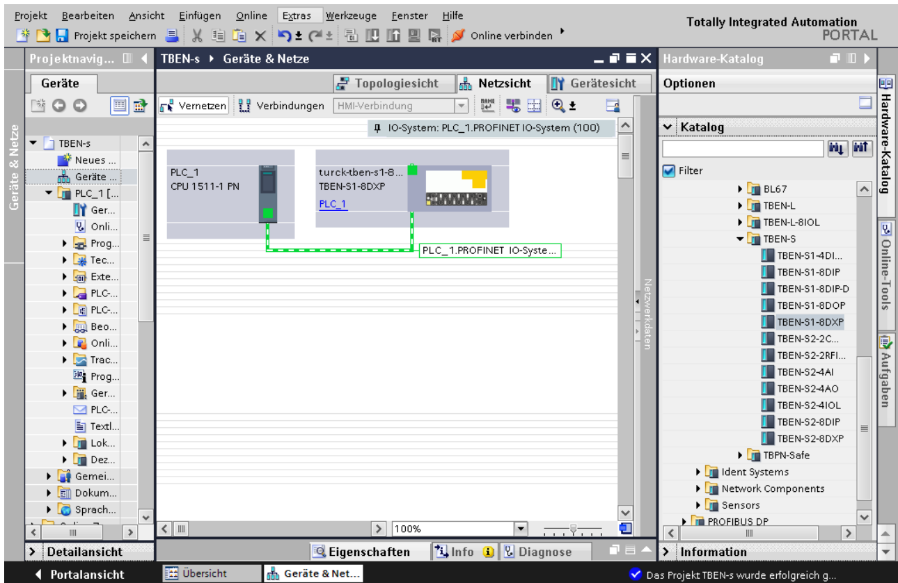
Abb. 46: Gerät mit der Steuerung verbinden
