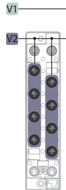
Abb. 25: Versorgung TBEN-S1-8DOP
