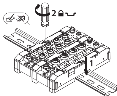
Abb. 11: Modulverbund auf Hutschiene montieren
