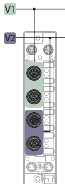
Abb. 28: Versorgung TBEN-S2-8DXP
