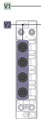
Abb. 30: Versorgung TBEN-S2-4AO
