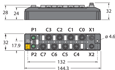
Abb. 1: TBEN-S1-... – Abmessungen
