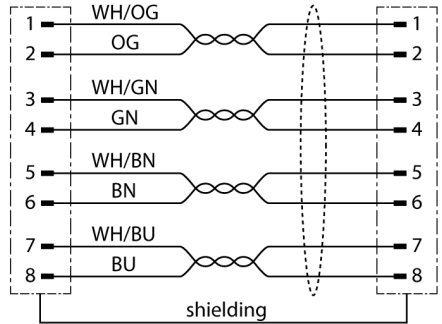
电路图
