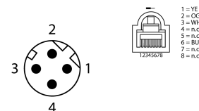
Schéma zapojení
