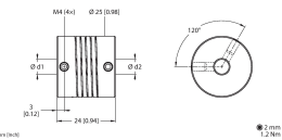
Wendelkupplung aus Aluminium Ø 25mm; d1=6mm, d2=10mm
