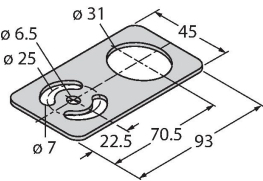
Montagewinkel, Edelstahl, für 30mm-Gewinde, Gewinde M10 x 1,5
