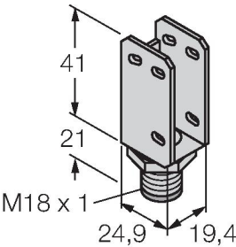
Montagewinkel, Edelstahl, für 18 mm Gewinde
