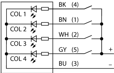
Anschlussbild
