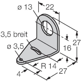
Montagewinkel, Werkstoff VA 1.4401, für Bauform QS12 & M12
