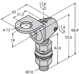
Montagewinkel, Edelstahl, für Bauform M12, Gewinde M10 x 1,5
