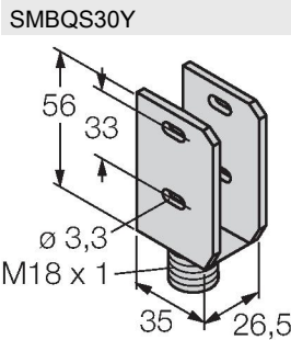
Schutzgehäuse, Edelstahl, für Bauform QS30
