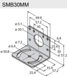
Montagewinkel, rechtwinklig, Edelstahl, für Sensoren mit 30 mm Gewinde, weite Bohrlöcher zur genauen Ausrichtung
