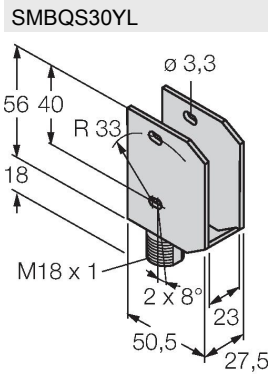
Schutzgehäuse, Edelstahl, für Bauform QS30
