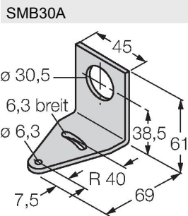
Montagewinkel, rechtwinklig, Edelstahl, für Sensoren mit 30mm Gewinde
