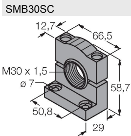
Montagewinkel, rechtwinklig, Edelstahl, für Sensoren mit 30 mm Gewinde, weite Bohrlöcher zur genauen Ausrichtung
