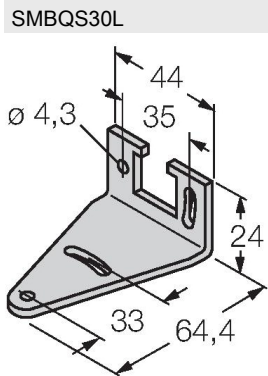
Montagewinkel, rechtwinklig, Edelstahl, für Sensoren mit 30mm Gewinde
