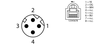
Schaltplan
