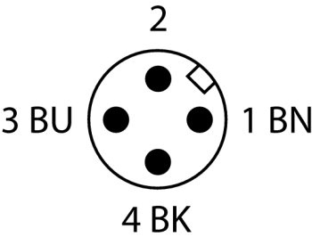
Schaltplan
