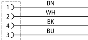
Schaltplan
