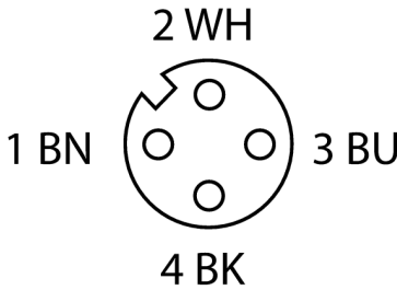
Schaltplan
