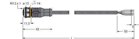
Dibujo acotado Tipo RKC4.4T-2/TEL N.º de ID 6625013
