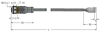
Dibujo acotado Tipo RKC4.5T-2/TEL N.º de ID 6625016
