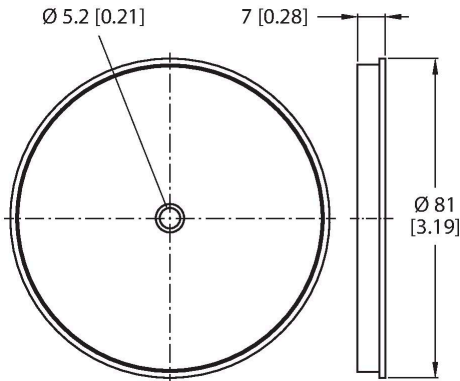
Dibujo acotado
