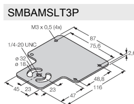
panel de montaje, acero inoxidable, para modelo LT3
