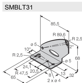
ángulo de montaje, acero inoxidable, para modelo LT3
