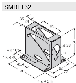
carcasa de protección, acero inoxidable, para modelo LT3
