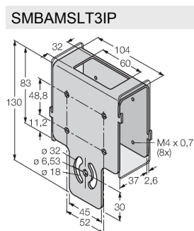
carcasa de protección con cristal protector, acero inoxidable, para modelo LT3
