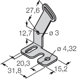
Dibujo acotado Tipo N.º de ID PKG4M-2/TEL 6625061
