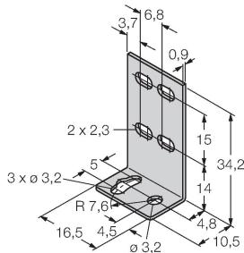
SMBQ12T
