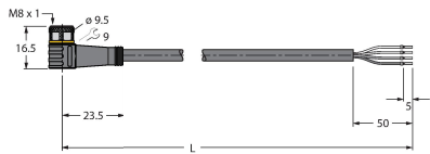
Dibujo acotado
