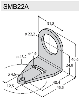
ángulo de montaje, acero inoxidable, para modelo K30L
