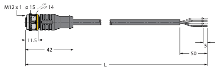
Dibujo acotado Tipo N.º de ID RKC4.4T-2/TEL 6625013
