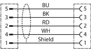
diagrama de conexiones
