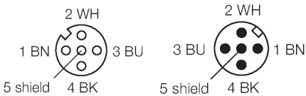
diagrama de conexiones
