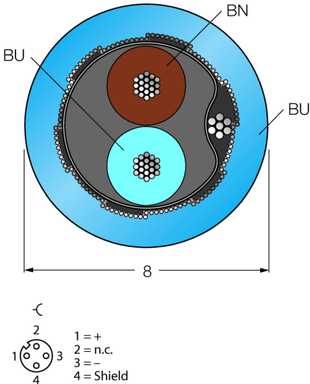
Sección transversal del cable
