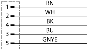
schéma de connexions
