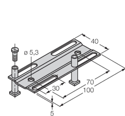
montage-instelrail voor rechthoekige bouwvorm CK40 / CP40; materiaal: VA 1.4301
