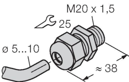
Kabelwartel M20 x 1,5
