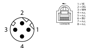
schakelplan
