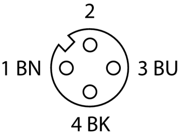
schakelplan
