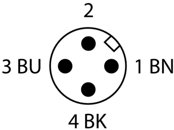
schakelplan
