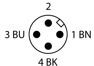
schakelplan
