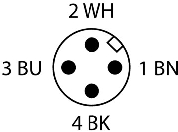
schakelplan
