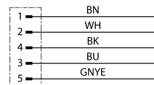
schakelplan
