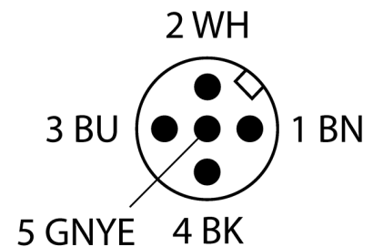
schakelplan
