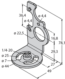
Uchwyt do montażu z lewej strony
