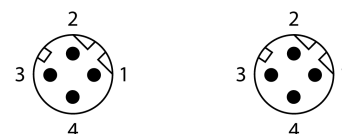
schemat obwodu
