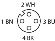
schemat obwodu
