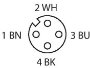
schemat obwodu
