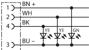
schemat obwodu
