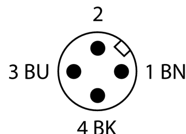
schemat obwodu
