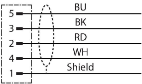
schemat obwodu
