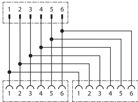
schemat obwodu
