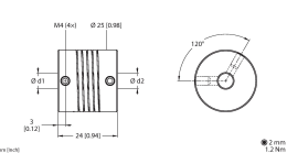
Cuplaj elicoidal din aluminiu Ø 25 mm; d1 = 10 mm, d2 = 12 mm
