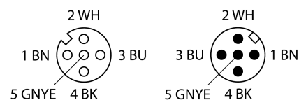
Schema de conexiuni
