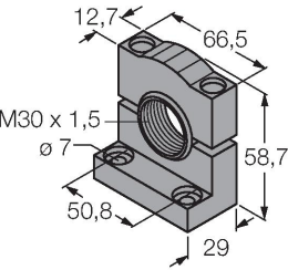
Монтажный зажим, РВТ черн., для датчиков с резьбой 30 мм, поворотный
