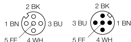
схема
