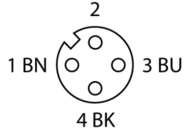
Devre şeması
