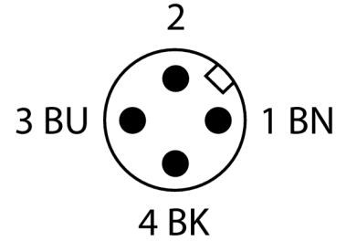
Devre şeması
