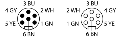
Devre şeması
